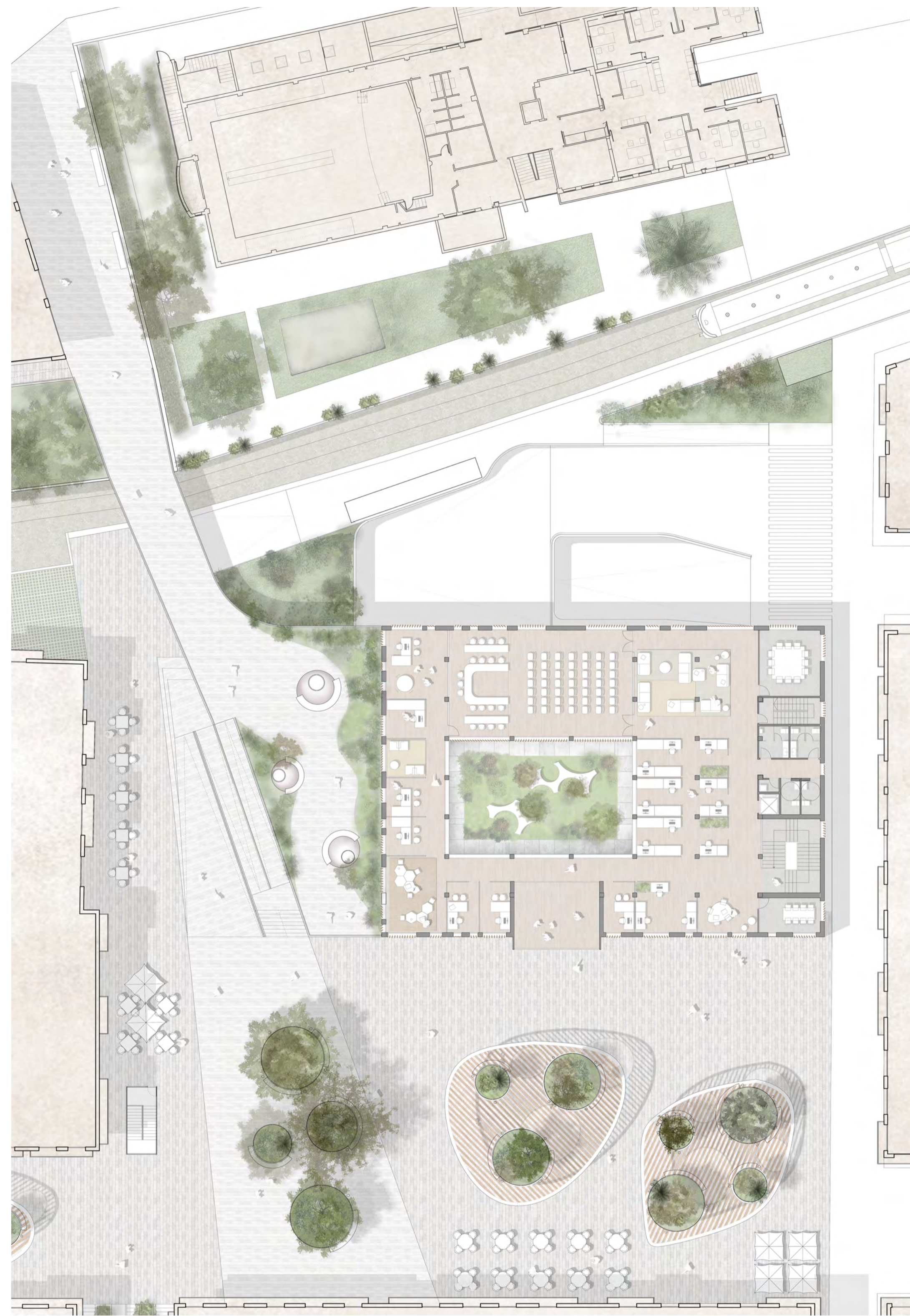
E: 1/250 0 1 5 10 15 20 25 PLANTA PRIMERA
